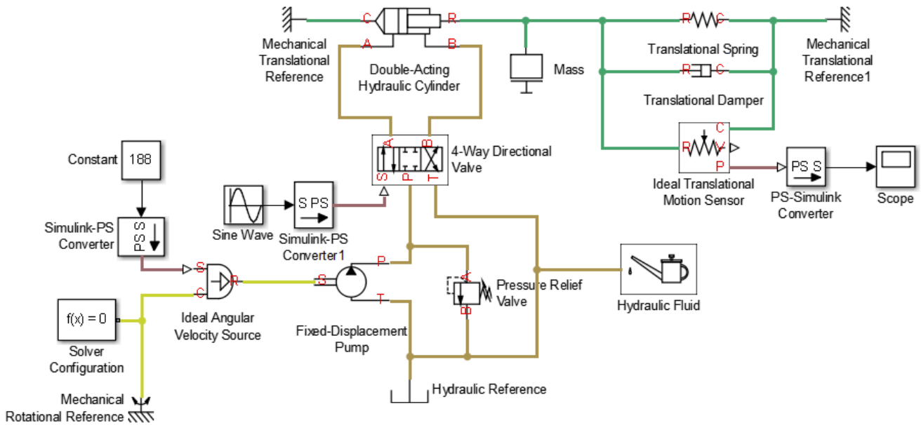
Рисунок Б.1 – Імітаційна модель автоматизованого гідропривода в програмному середовищі SimScape
